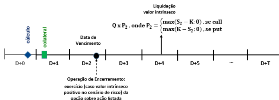
Figura 7.42 - Encerramento de posição comprada, com vencimento próximo, em opção listada sobre ação
