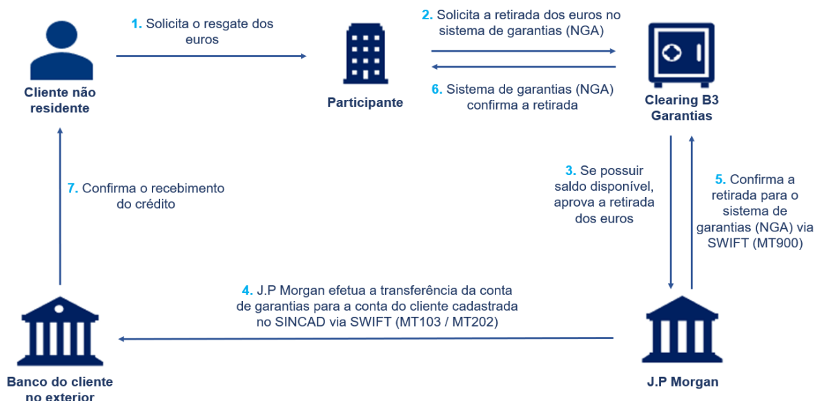
Figura 19. Fluxo de retirada de euros para a conta do cliente
