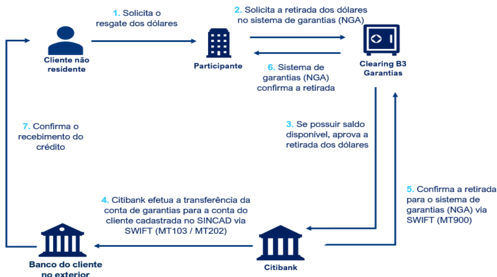
Figura 16. Fluxo de retirada de dólares para a conta do cliente
